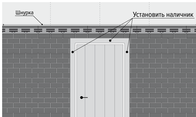
Рис. 16. Установка наличников
